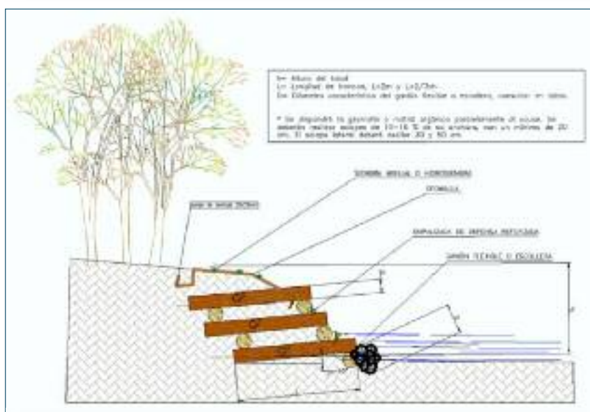
Figura 6.14 Croquis de una ficha de ejecución de técnica de bioingeniería
